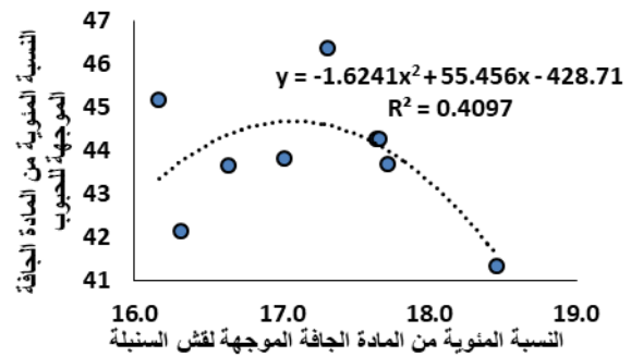
شكل (5) علاقة الانحدار بين % من المادة الجافة الموجهة لقش السنبلة و% من المادة الجافة الموجهة للحبوب لمجموعة من الأنماط الوراثية للقمح الصلب
